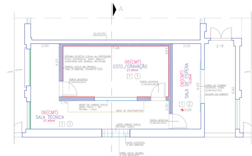
Planta baixa do estúdio multifuncional, localizado na Central de Aulas
